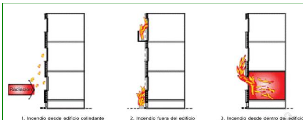
Figura 1. Mecanismo de propagación del fuego en fachadas. Fuente: Kotthoff y Riemesch.
